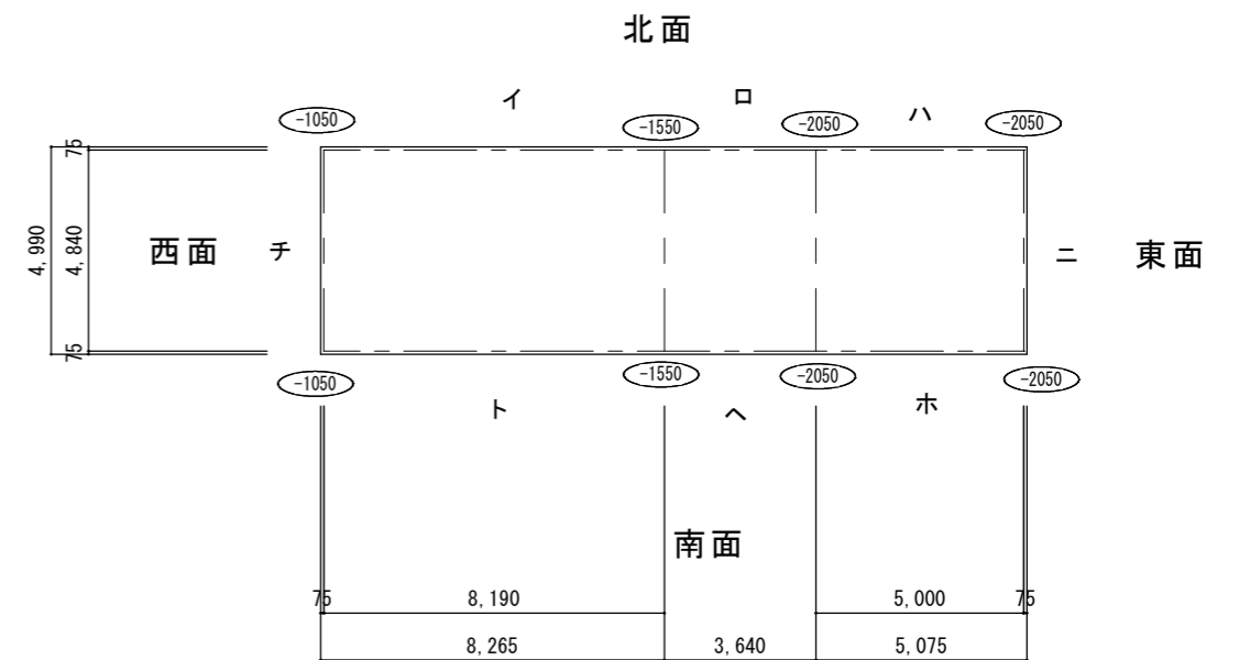
地盤面算定図 S=1/200
